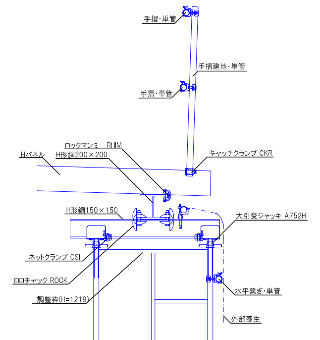
断面詳細図(水下)
