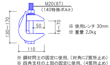
ロコチャック(形状・寸法)
