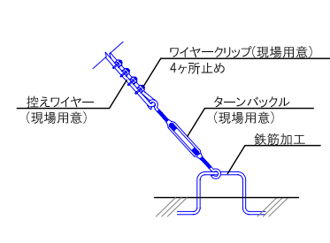
控えワイヤー詳細図(躯体側)
