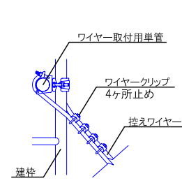
控えワイヤー詳細図(建柱)
