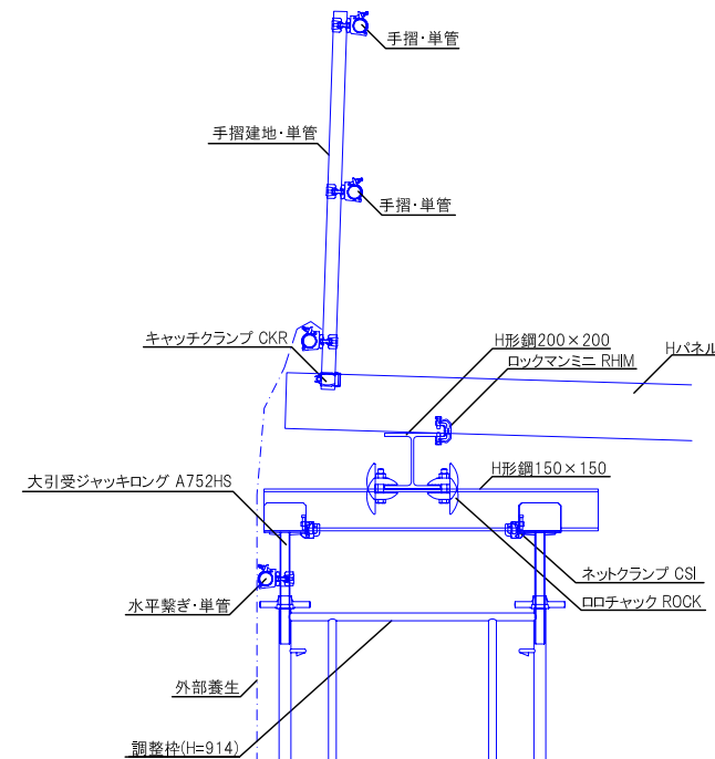
断面詳細図(水上)
