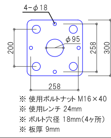
四角支柱(形状・寸法)
