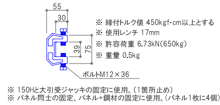
ロックマンミニ(形状・寸法)
