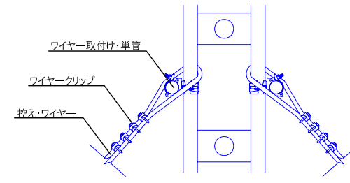
控えワイヤー詳細図(四角支柱)
