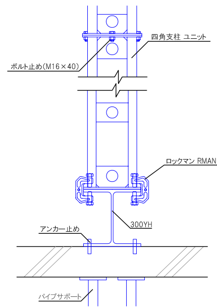
四角支柱脚部詳細図
