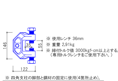
ロックマン(形状・寸法)
