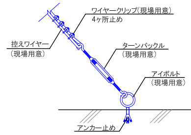
控えワイヤー詳細図(躯体側)
