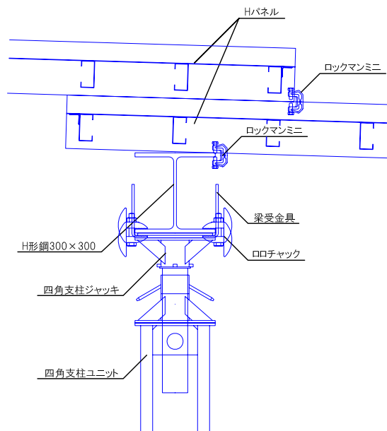
四角支柱上部詳細図
