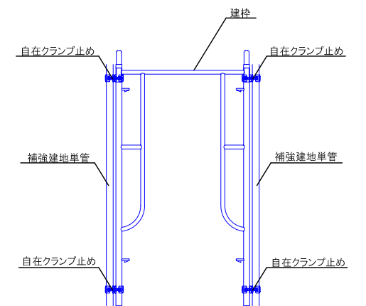
建柱補強詳細図
