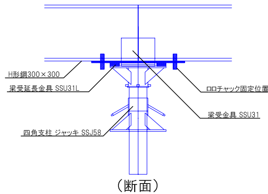
桁材継ぎ部分詳細図(1本受け)
